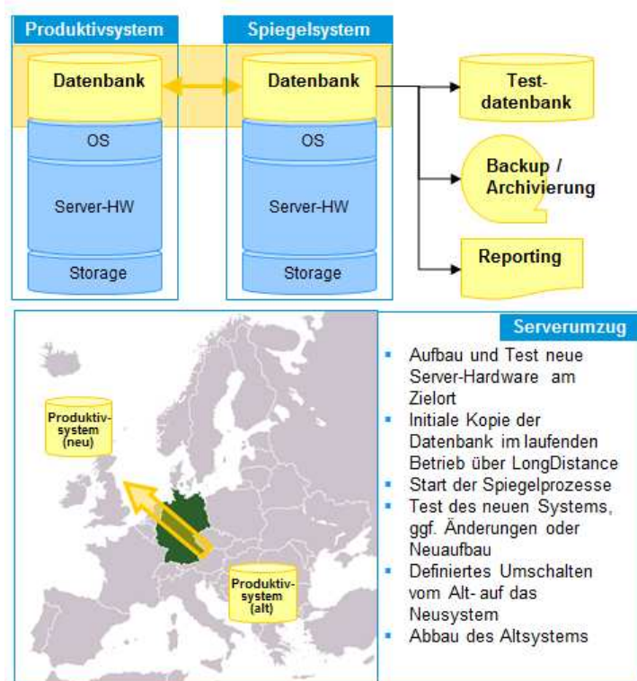
Abb. 1: Zusatznutzen Standby-System
