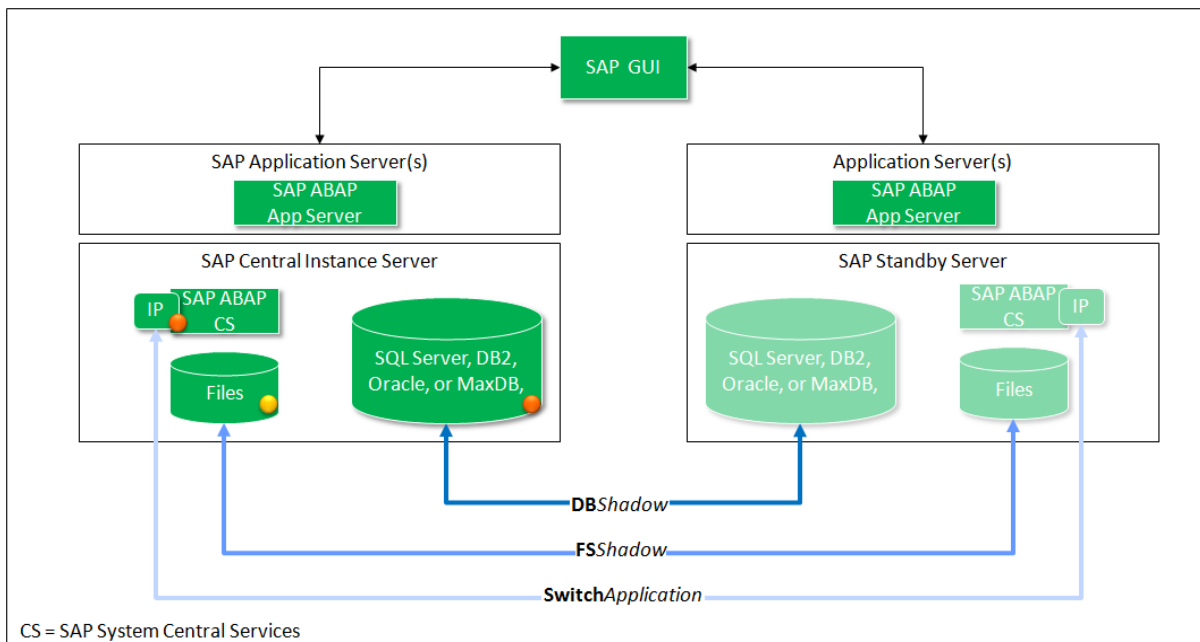
Abb. 3: Absicherung SAP-ABAP-Datenbank
