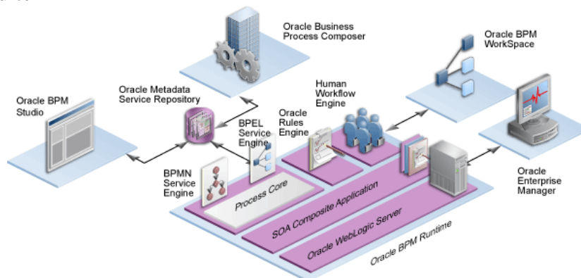
Abb. 3: BPM Komponenten
