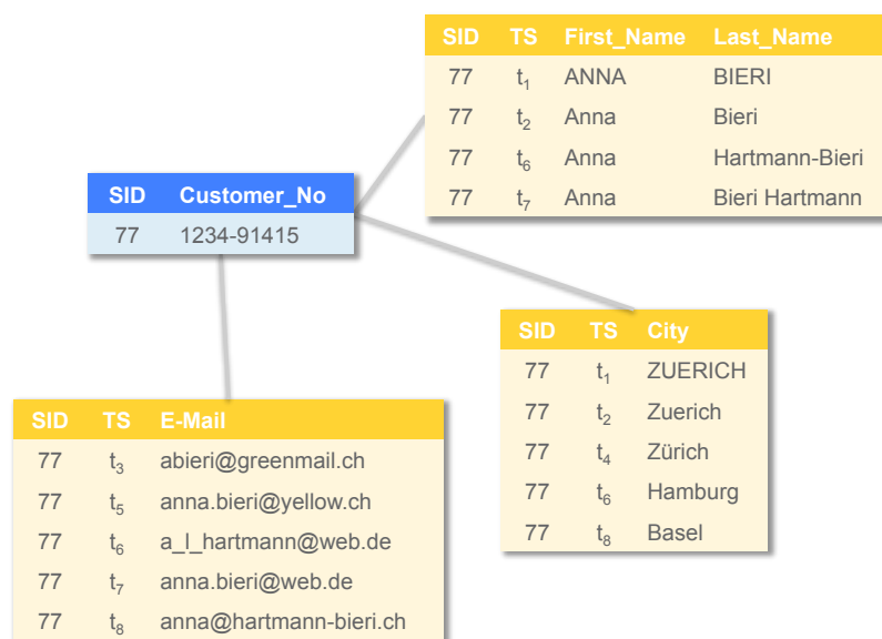
Abbildung 3: Historisierung von Kundendaten in den Satelliten
