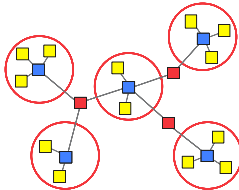
Abbildung 1: Grundprinzip von Data Vault mit Hubs (blau), Links (rot) und Satellites (gelb)
