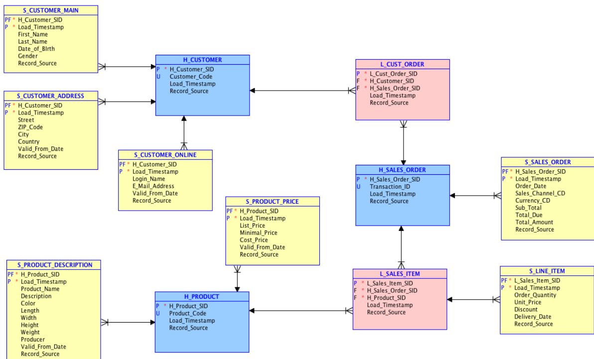
Abbildung 2: Beispiel für ein Data Vault Modell
